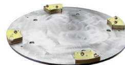
Skiva med PCD-knappar för avverkning av mattreser och andra ytbeläggningar
