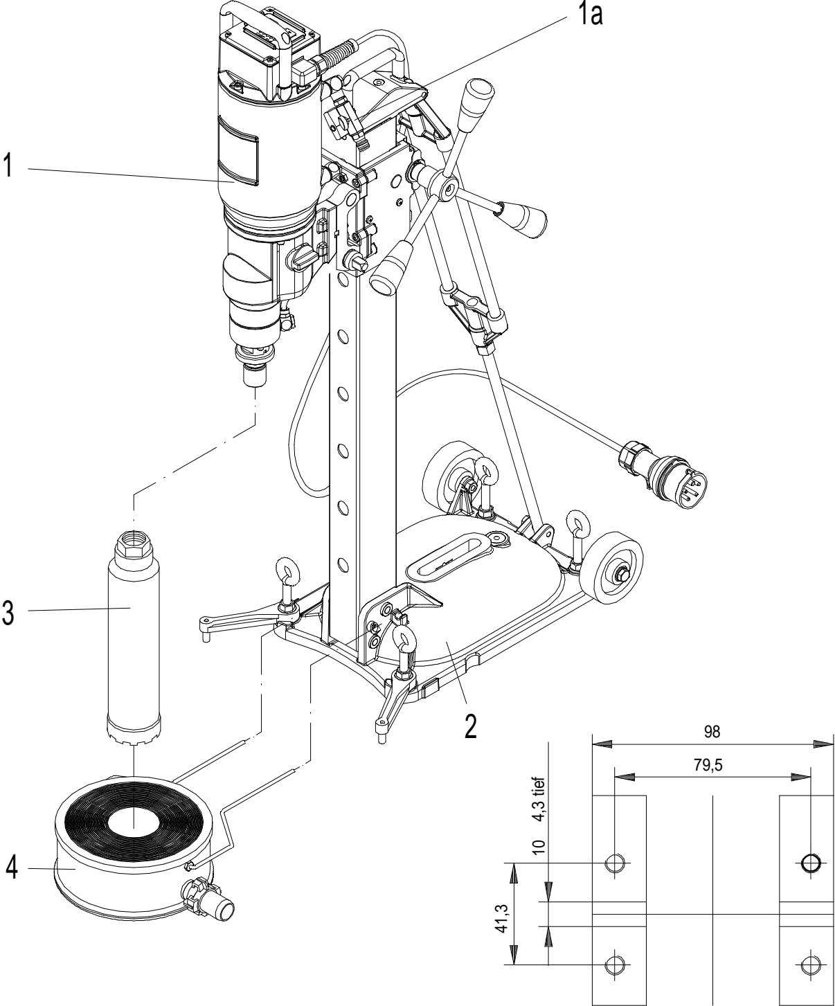
Maße - Getriebefuß
