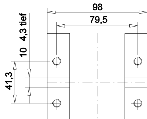
Maße - Getriebefuß
